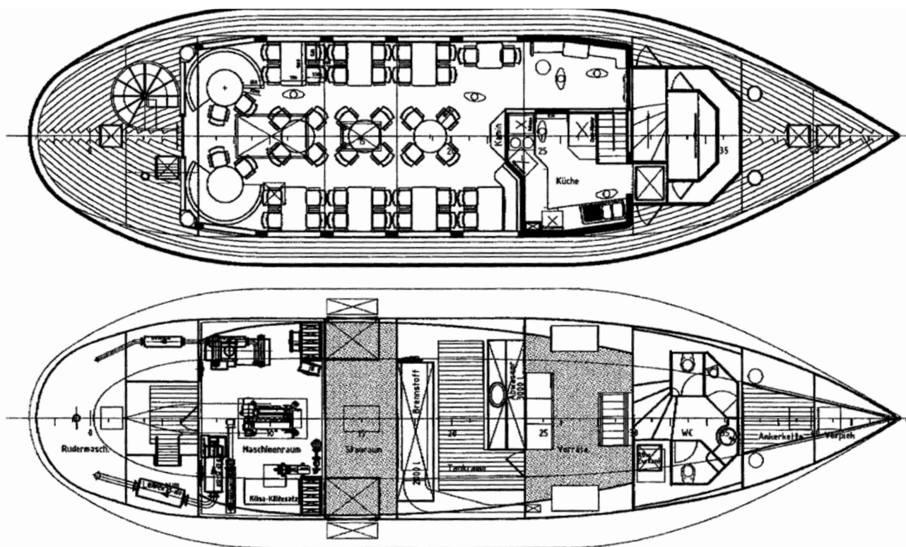
Grundriss der M.Y. «Emily»
