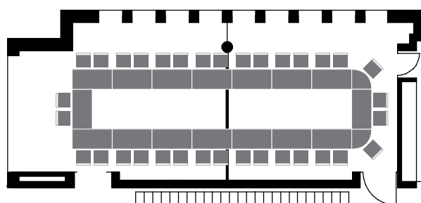
U-Bestuhlung 34 Sitzplätze
