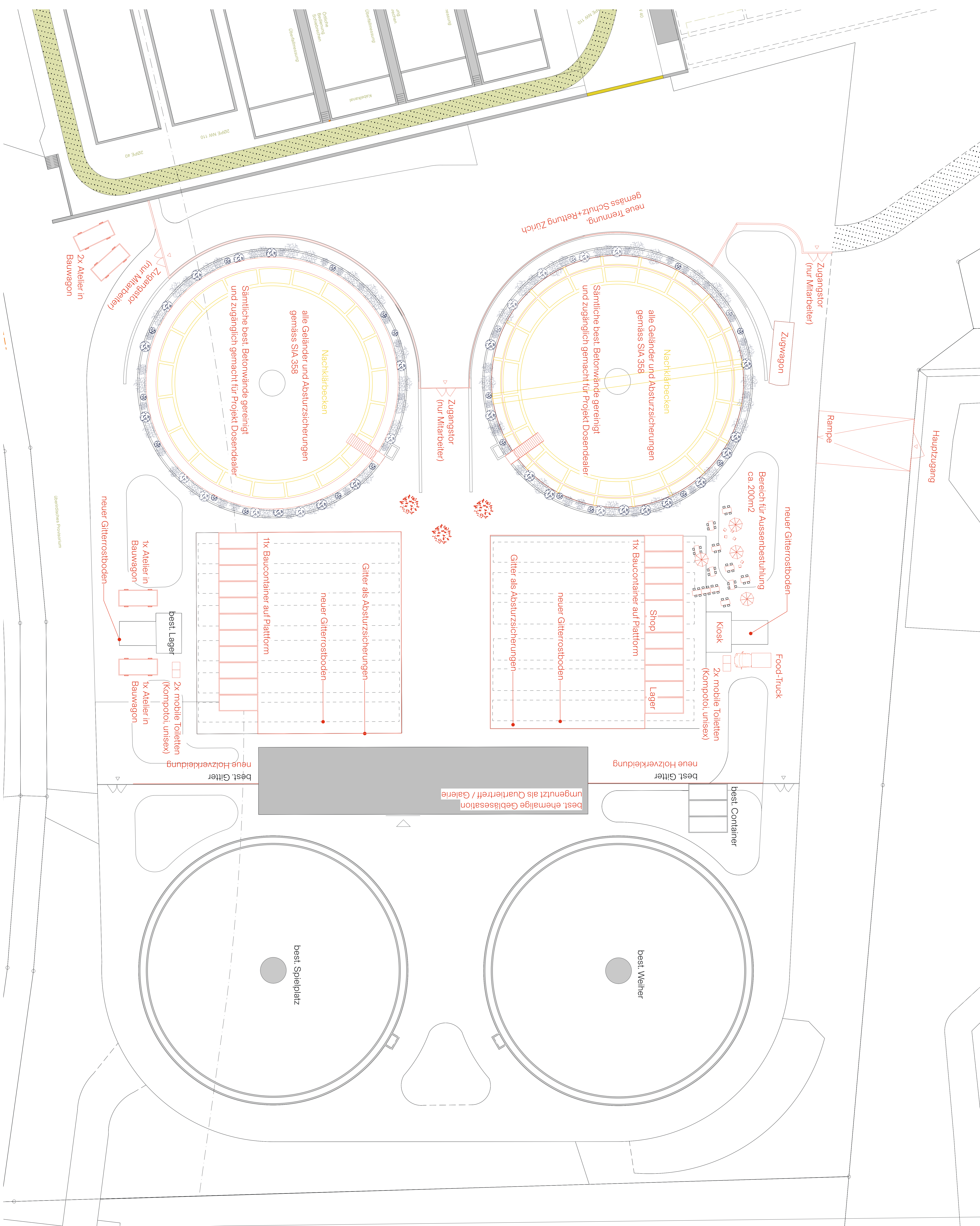
Umgebungsplan Gesamtanlage, Mst. 1:500
